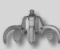
Mehrschalengreifer
