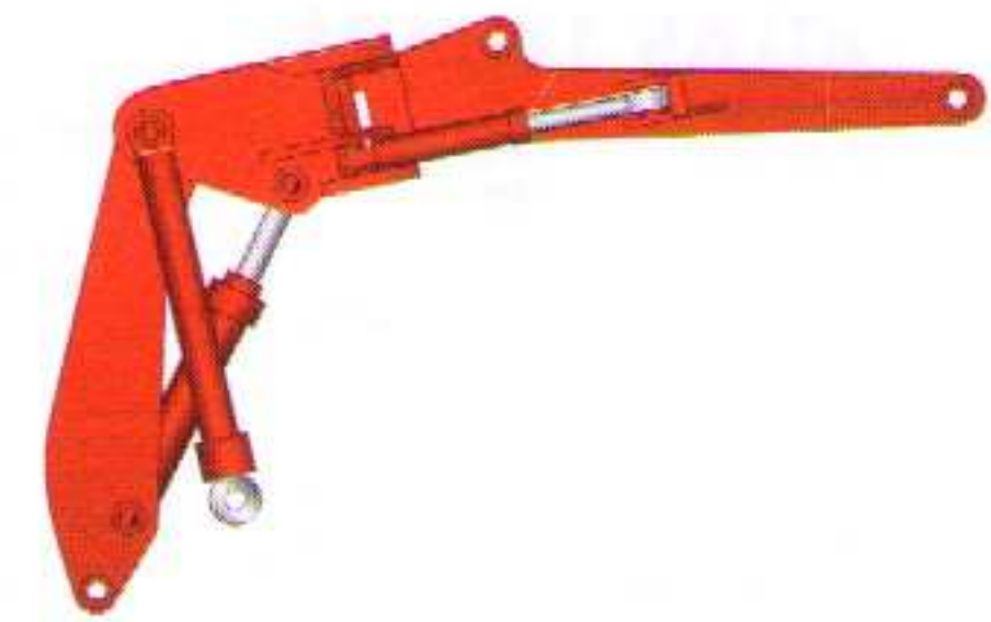
Grundarm C 53.41 mit Ausleger C 43.47 Nutzlänge 3350 mm
