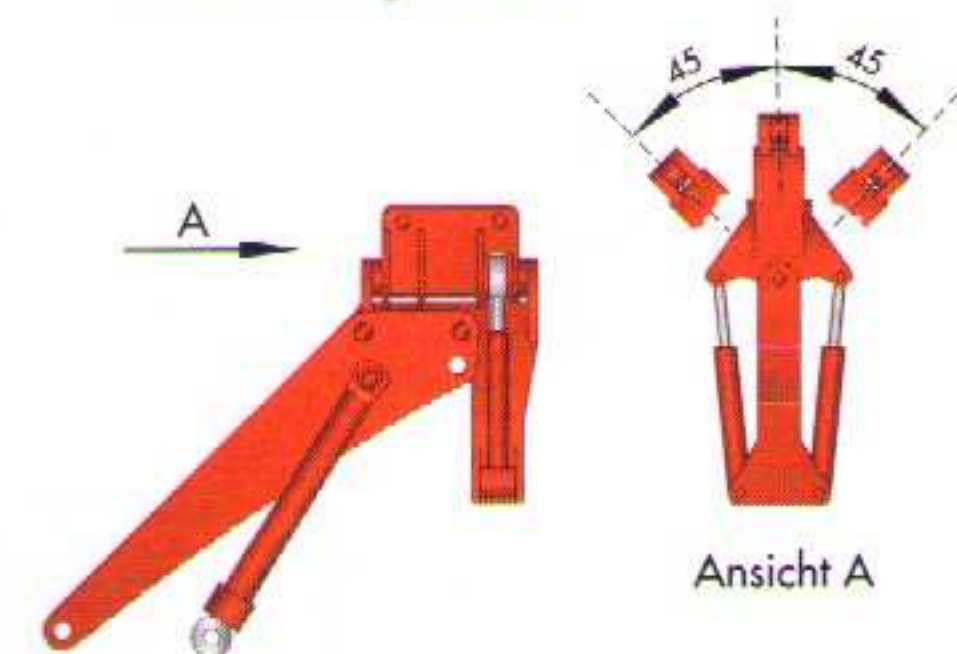
Grundarm C 53.0 mit verstellbarem Gelenk C 53.9 mit 2 Zylindern
