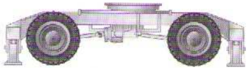
Grundgerät A 43.32 4-fache Prattenabstützung, hydraulischer Verstellarm
